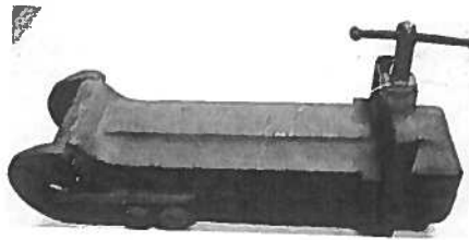
Jernstøbeform til to tene fra 1800-tallet. Formen ligger ned på illustrationen. Toppens/åbningen er i enden til højre. Håndtaget løsnes og trækkes op over åbningen, når formen skal åbnes. Fra Mønten i København. Nu hos Danmarks Tekniske Museum, Helsingør.
